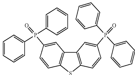
PPT
