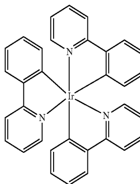
Ir(ppy) 3
